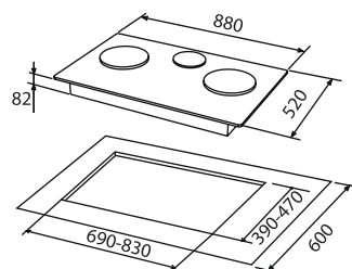
GAS HOB / FH-GS3030 SVGL
