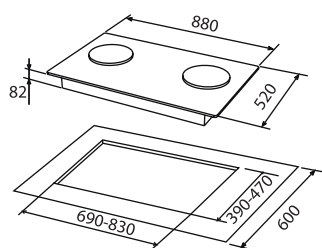
GAS HOB / FH-GS3028 SVGL
