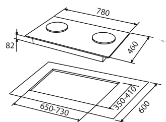
GAS HOB / FH-GS3020 SVGL
